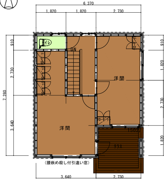
2階平面図
