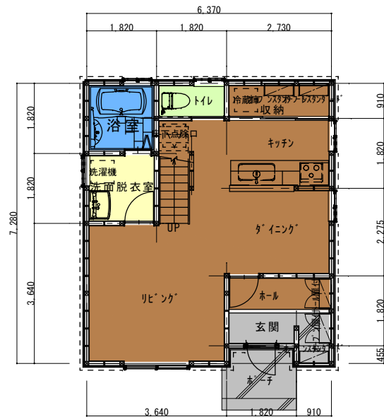
1階平面図
